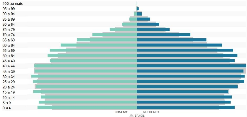
Pirâmide Etária - 2022
